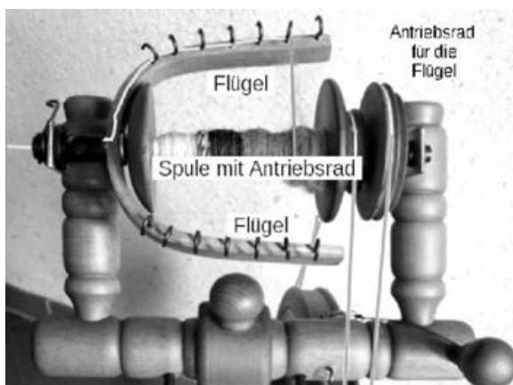
Bild 26: Details: Spule und Flügel
